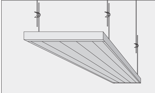
Figur 7. Atrium frihängande med panelhake och justerbara trådpendlar.
