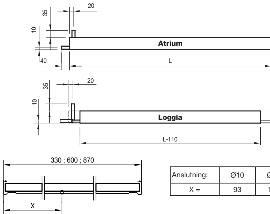
Figur 4.b. Atrium och Loggia mått, vatteninkoppling & anslutning.
