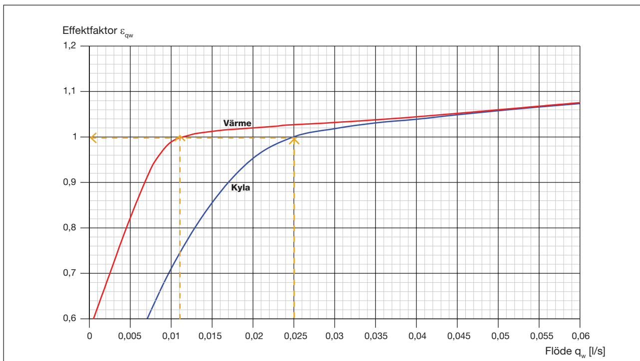
Diagram 3. Effektfaktor \epsilon_{qw} som funktion av vattenflöde q_w .
