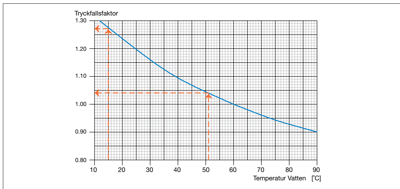
Diagram 7. Temperaturjusterad tryckfallsfaktor.
