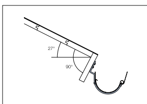
Lindab krok K11
