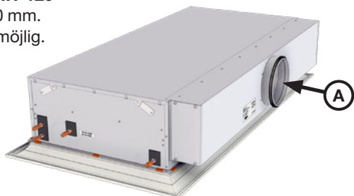
Bild 20. Möjliga Plexus tilluftanslutningar.
