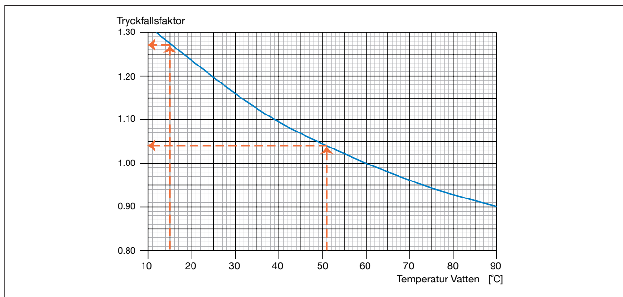
Diagram 7. Temperaturjusterad tryckfallsfaktor.
