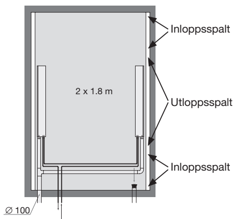
Figur 1. Två Celo bafflar med två öppna spalter.
