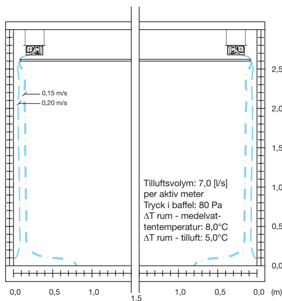
Figur 11 - 14. Lufthastigheter, heltäckande undertak med spalter längst väggar.
