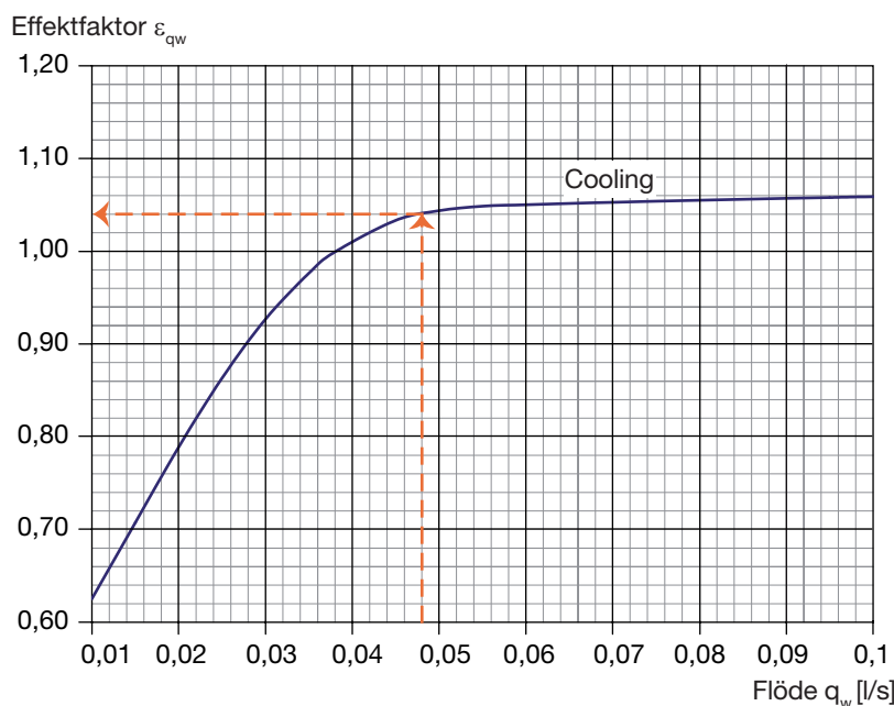
Diagram 3. Effektfaktor \varepsilon_{qw} som funktion av vattenflöde.
