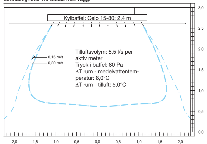
Lufthastigheter vid utblås mot vägg.
