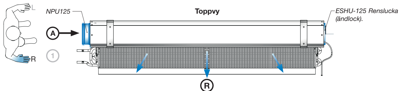
Bild 74. Konfiguration A1R: Tilluften tillförs rummet i riktning höger.
