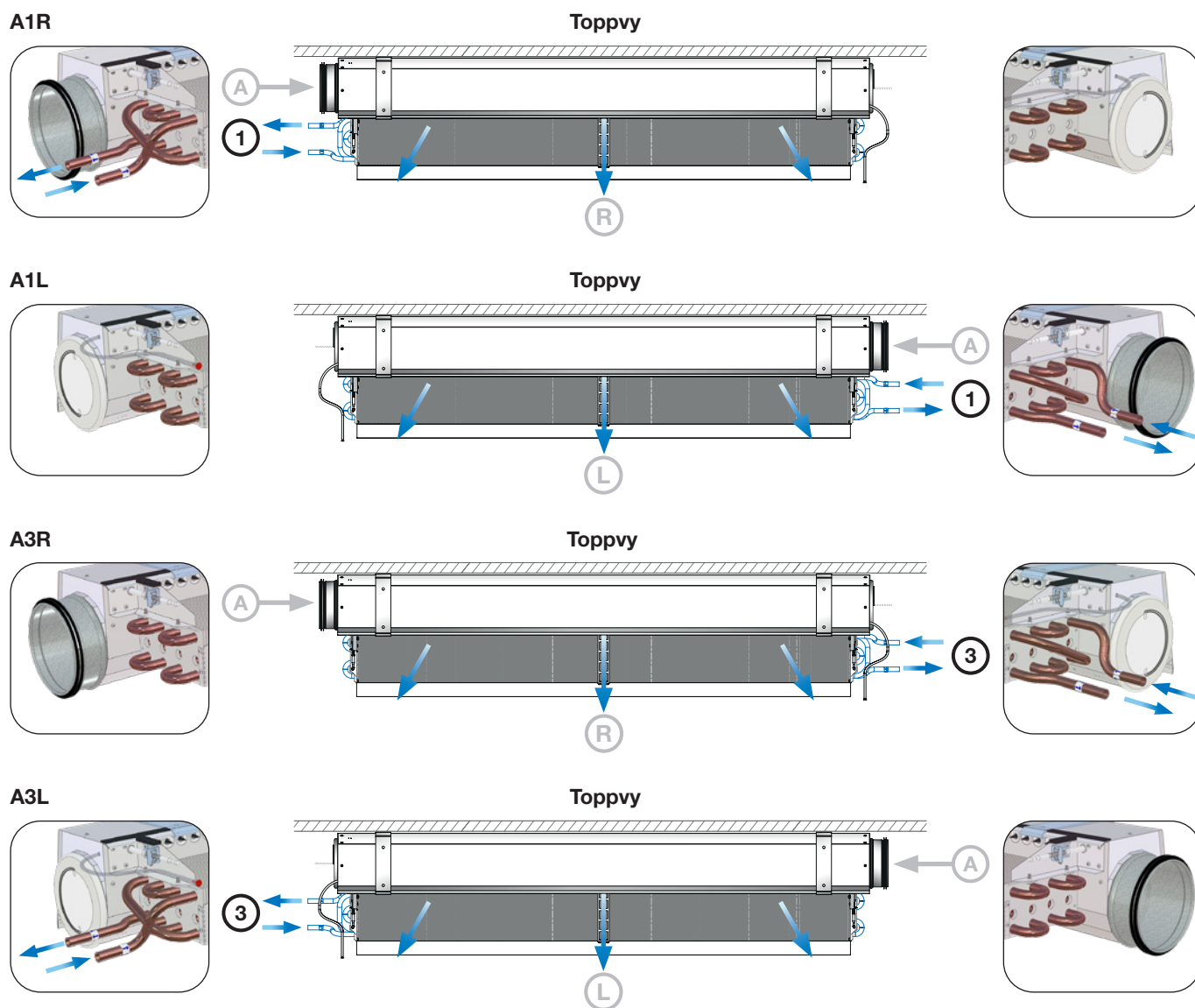
Bild 77. Beskrivning av vattenanslutningar för 2-vägs vattenkrets.
