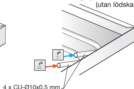
C7: Anslutningstyp 7: Snedställd (utan lödskarv)
