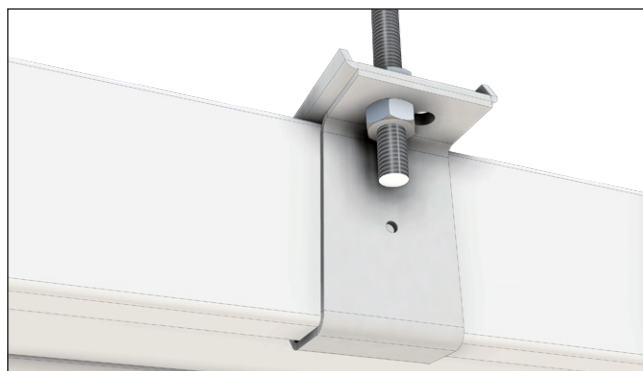
Figur 6. Atrium Säkerhets beslag för upphängning i idrotts-hallar (används för synlig fri upphängning i kombination med gångstänger).
