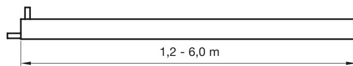
Figur 4. Atrium och Loggia tillverkas som standard i längd mellan 1,2 m till 6,0 m i steg om 0,1 m. Verkligt längdmått är -12 mm.
