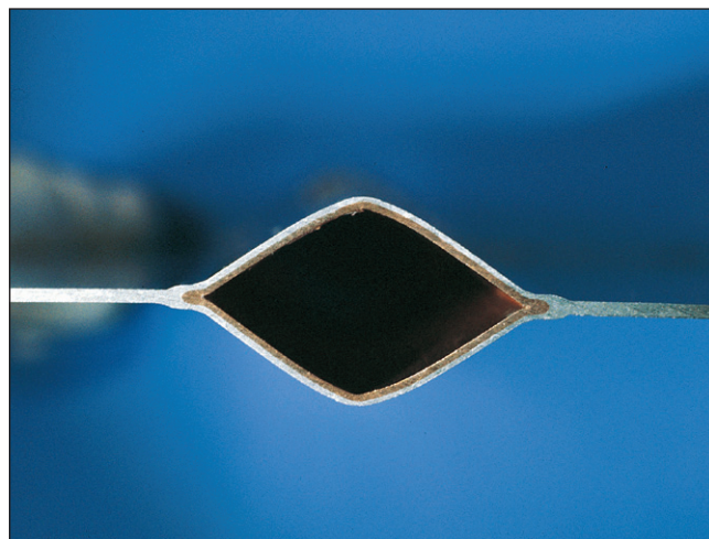
Bild 1. Visar ett tvärsnitt av koppar- och aluminiumplåtarna metallurgiskt förbundna samt den rombiskt formade vattenkanalen.
