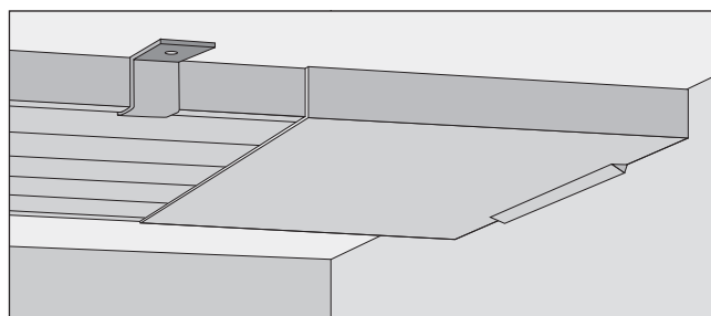
Figur 1. Atrium med anslutningskåpa. (ATR-CW).
