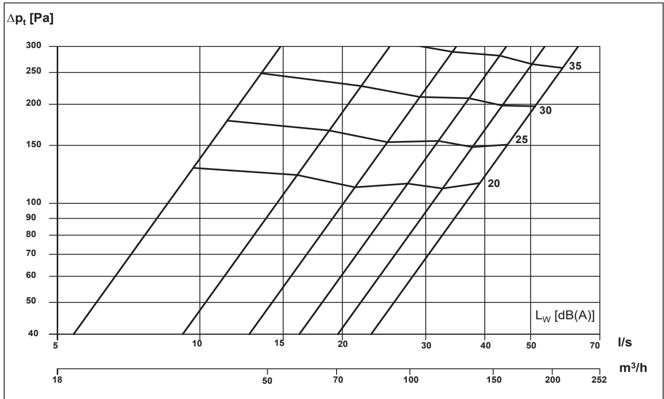
Diagram 9. Ljudeffektnivå L_w för \varnothing 200 anslutning.
