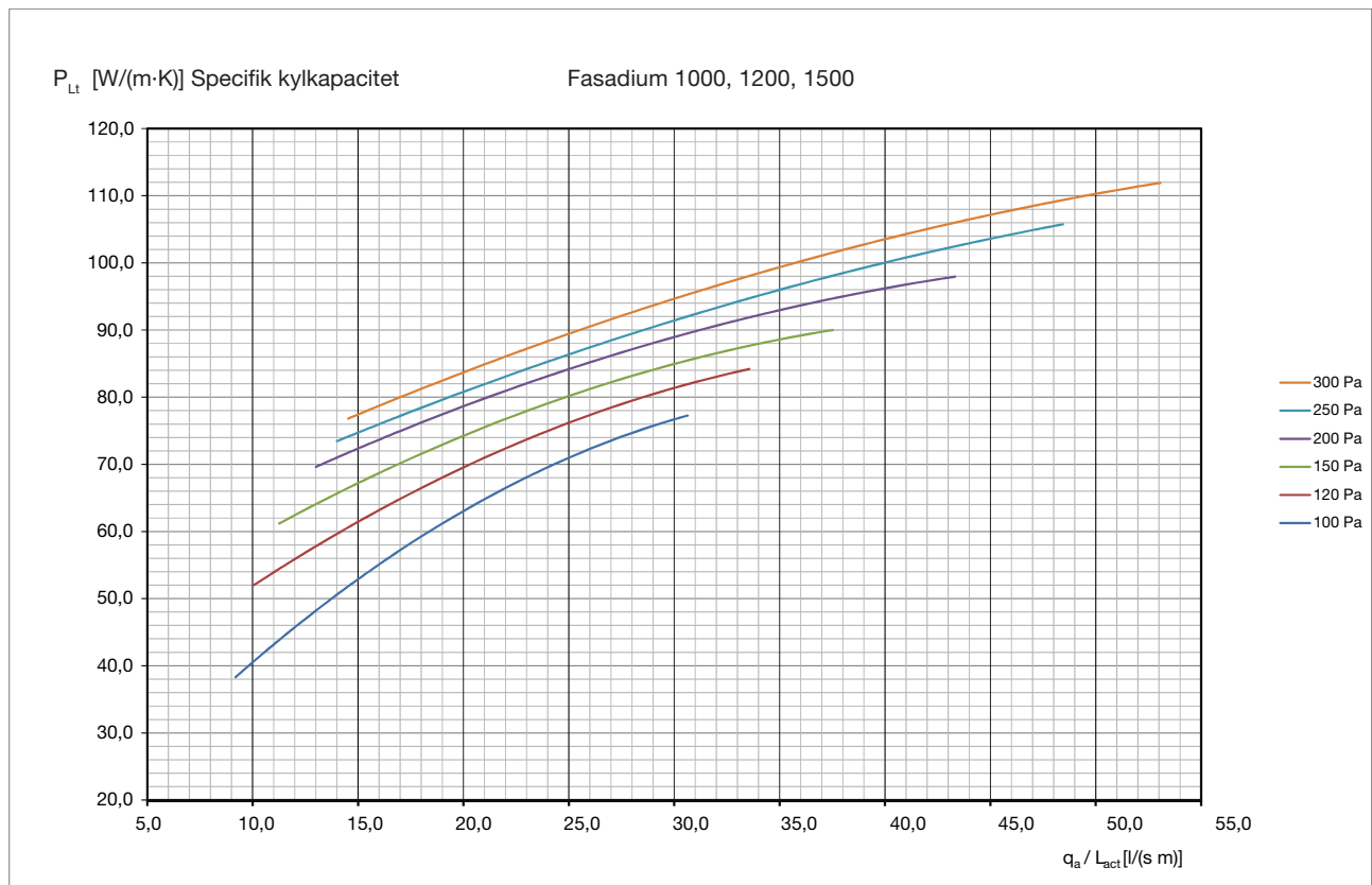
Diagram 3. Fasadium 1000, 1200, 1500: Specifik kylkapacitet P_{L_t} per aktiv meter och Kelvin som funktion av luftflöde per aktiv meter.
