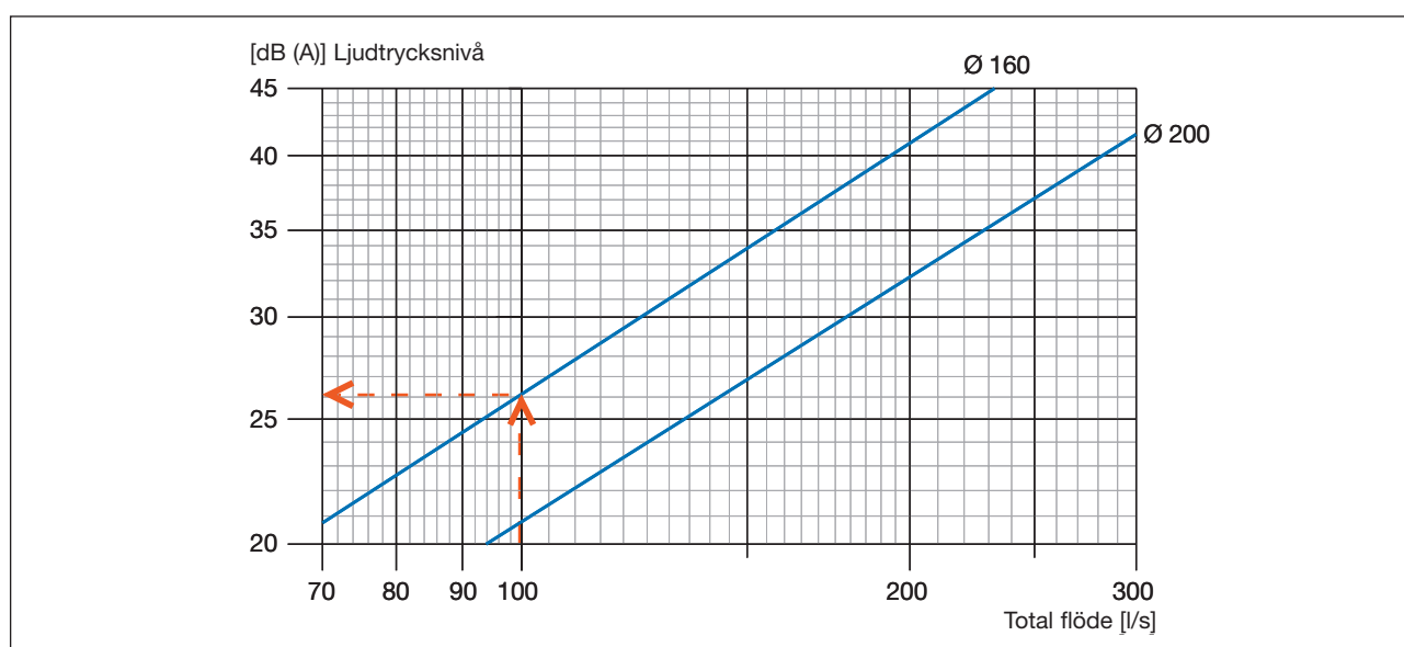
Diagram 10. Egenljudsalstring i första apparat. Ljudtrycksnivå med 10 m² Sabine rumsdämpning.
