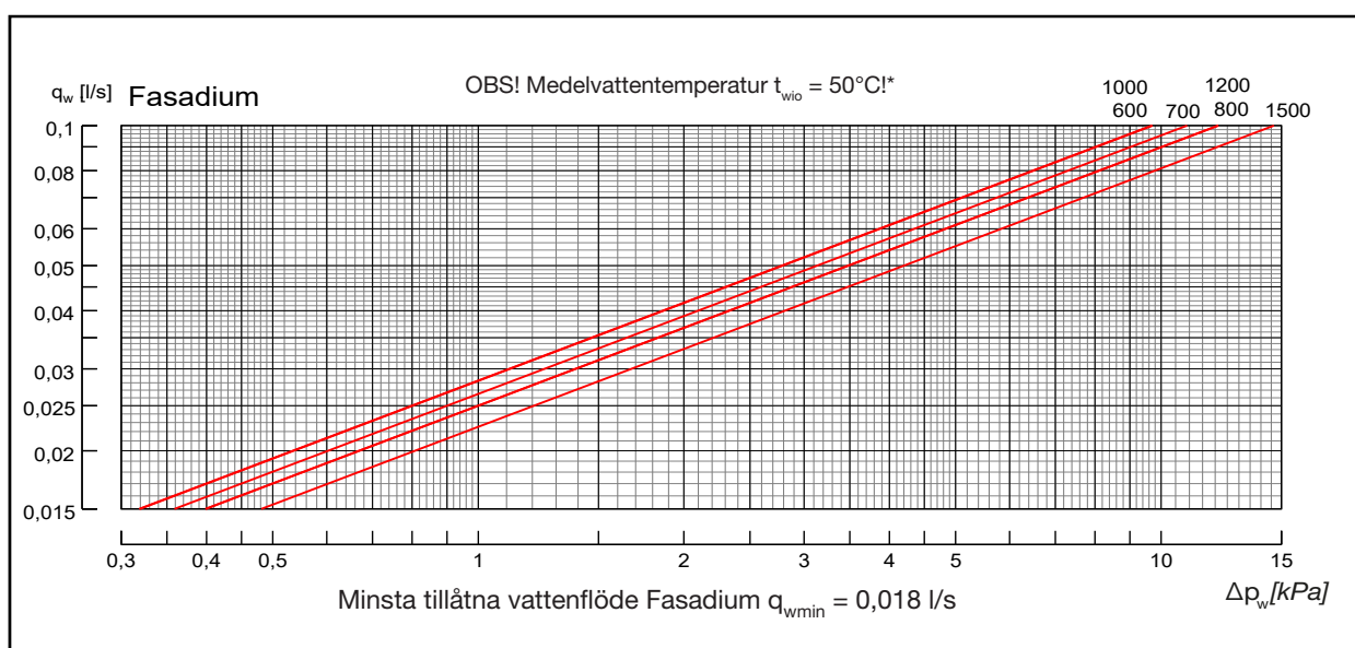
Diagram 13. Tryckfall i batteriets värmekrets.
