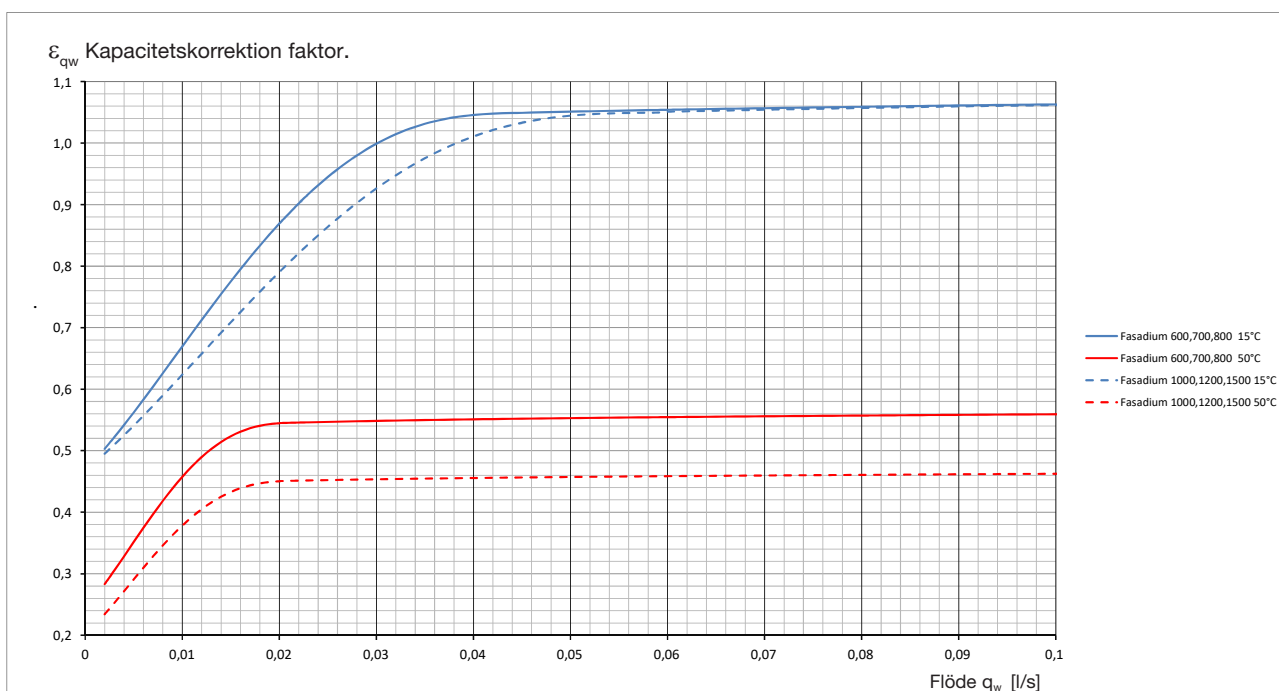
Diagram 5. Kapacitetskorrektion \varepsilon_{q_w} för vattenkretsen, både för kyla och värme.
