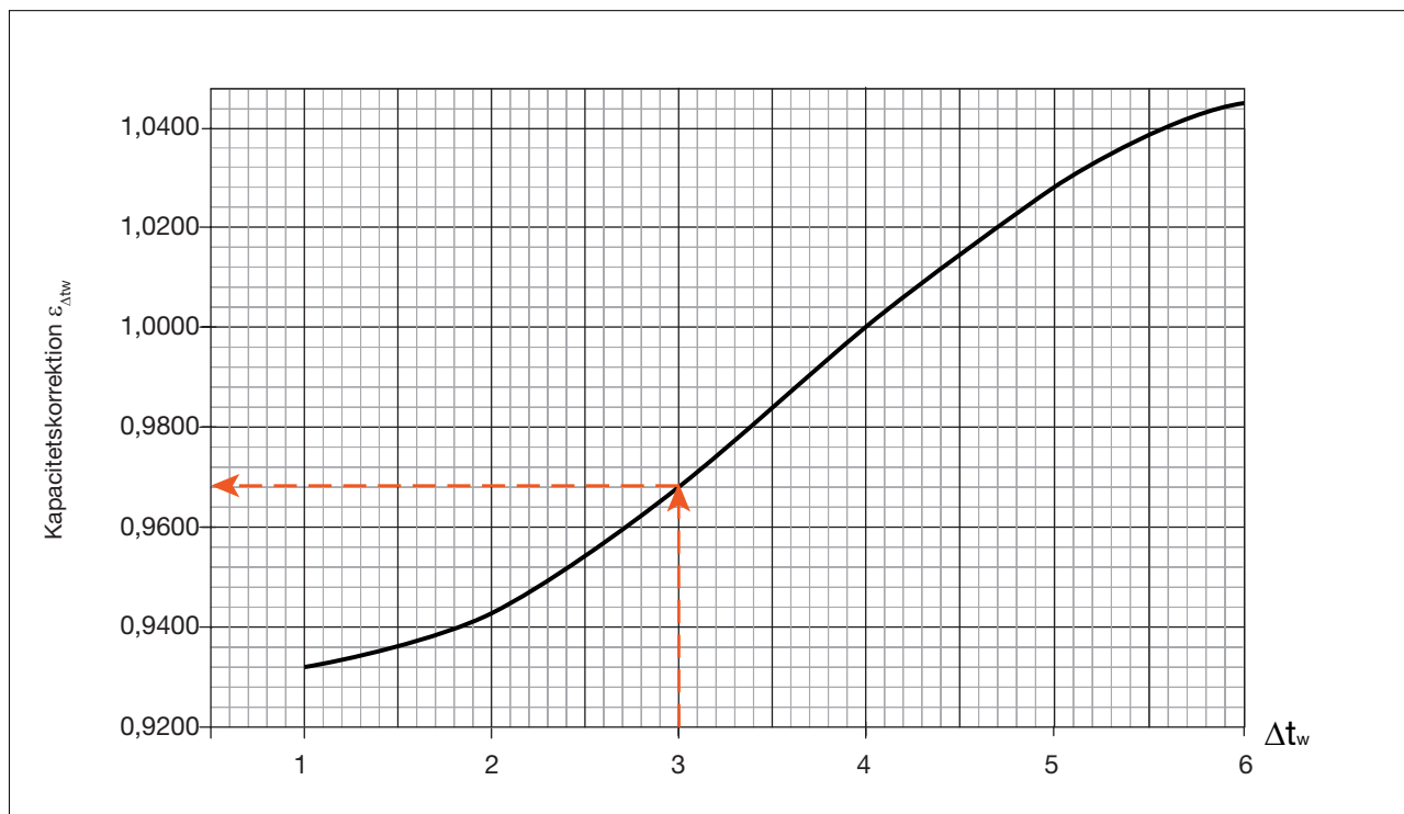
Diagram 4. Kapacitetskorrektion \varepsilon_{\Delta t_w} som funktion av vattenflödet \Delta t_w . Används enbart för kyla.
