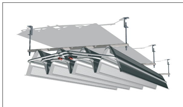
Bild 10. Montage av Carat med gängstänger.
