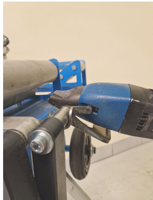
4. Montera plåtsax TRC200 på adaptern.
