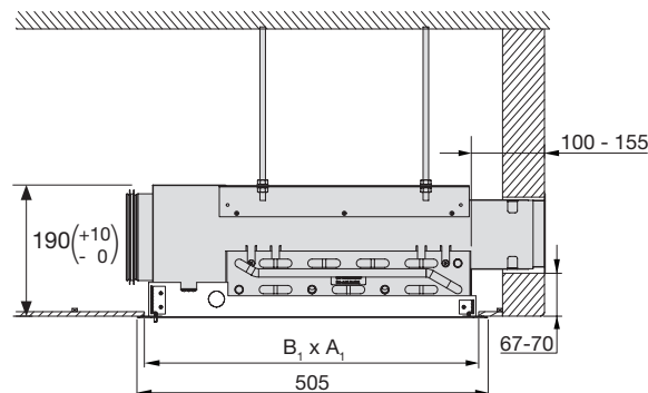
Figur 15. Installationsritning för frontplatta (inlopp) -03 och -3E med öppningsmått.
