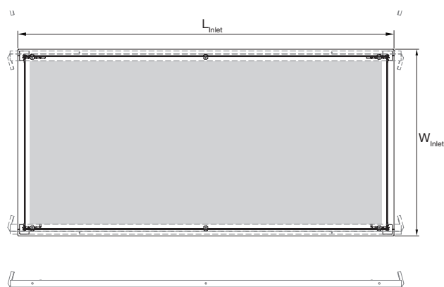
Figur 13. Mått för frontplatta (inlopp) -3L.
