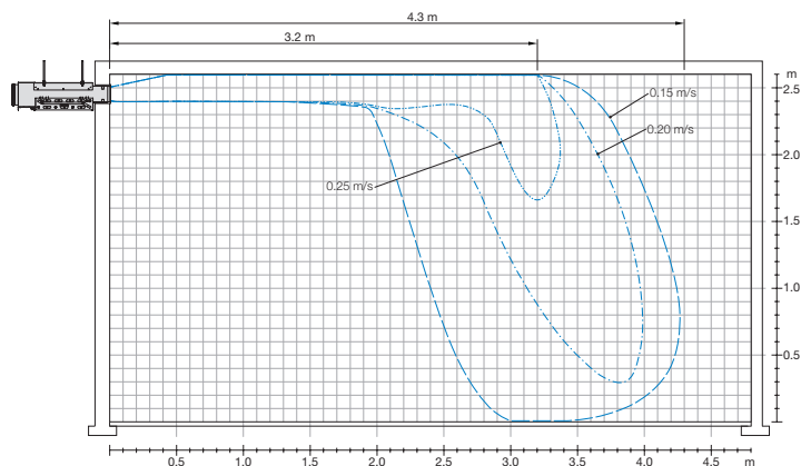
Figur 3: Sidovy B-B: Lufthastigheter för standard spridningsbild (30° - 0° - 30°).
