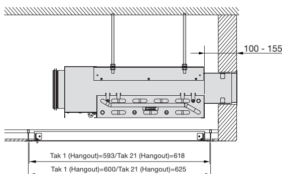
Figur 17. Installationsritning för frontplatta (inlopp) -01/-21 med utvändiga mått.
