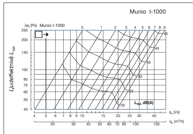
Diagram 6.b. Ljudeffektnivå L_{WA} Munio I-1000.
