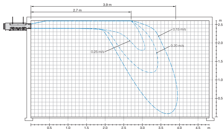
Figur 2: Sidovy A-A: Lufthastigheter för standard spridningsbild (30° - 0° - 30°).
