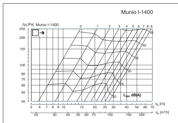
Diagram 6.d. Ljudeffektnivå L_{WA} Munio I-1400.
