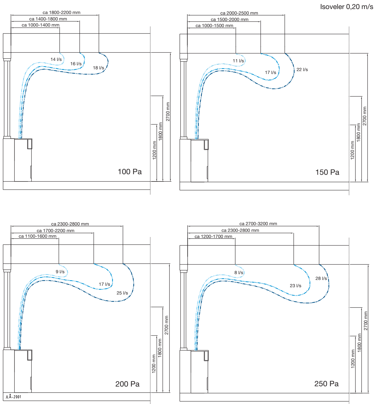
Figur 5. Fasadium - 800, spridningsbilder vid olika inställningar av luft och flöde.
