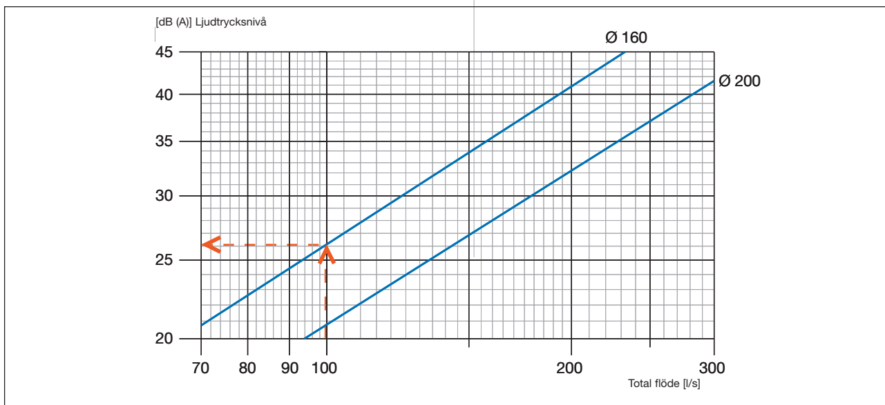
Diagram 10. Egenljudsalstring i första apparat. Ljudtrycksnivå med 10 m 2 Sabine rumsdämpning.
